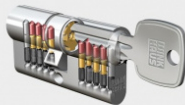
Cylindrická vložka Winkhaus - XR - třída 3
