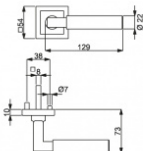
Cylindrická rukojeť
