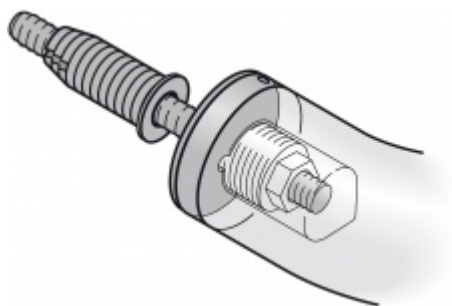
Skryté upevnění madla FSB 05 0580 00435 M6
