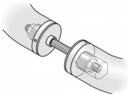
Párové propojení madla 05 0580 M8
